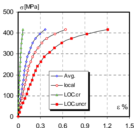
Slika 1. Zavisnost napon-deformacija TP1 Figure 1. Stress-strain diagram TP1.
